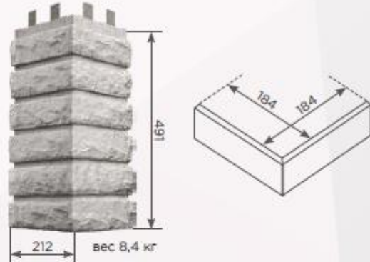
УГОЛ НАКЛАДНОЙ
