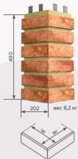
УГОЛ НАКЛАДНОЙ
