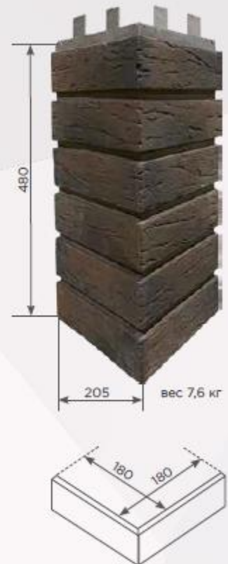
УГОЛ НАКЛАДНОЙ
