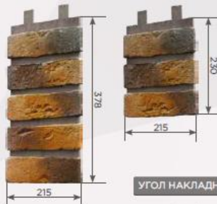
ОБРАМЛЕНИЕ ВЫСОТОЙ 3 И 5 КИРПИЧА
