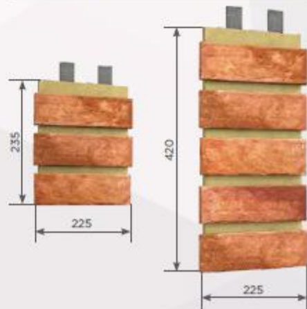
ОБРАМЛЕНИЕ ВЫСОТОЙ 3 И 5 КИРПИЧА
