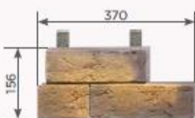
УГОЛ СОСТАВНОЙ ПРАВЫЙ
